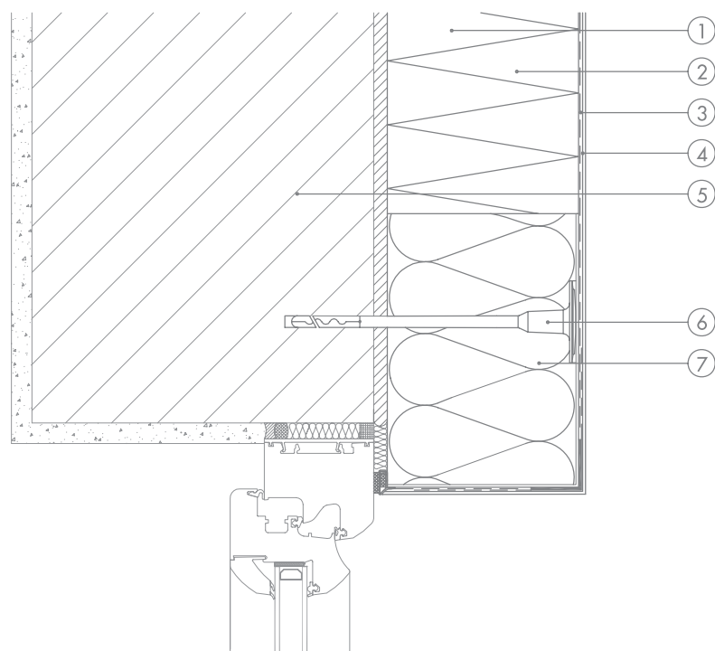
b) kod prozora postavljenog u ravnini s vanjskim rubom zida
