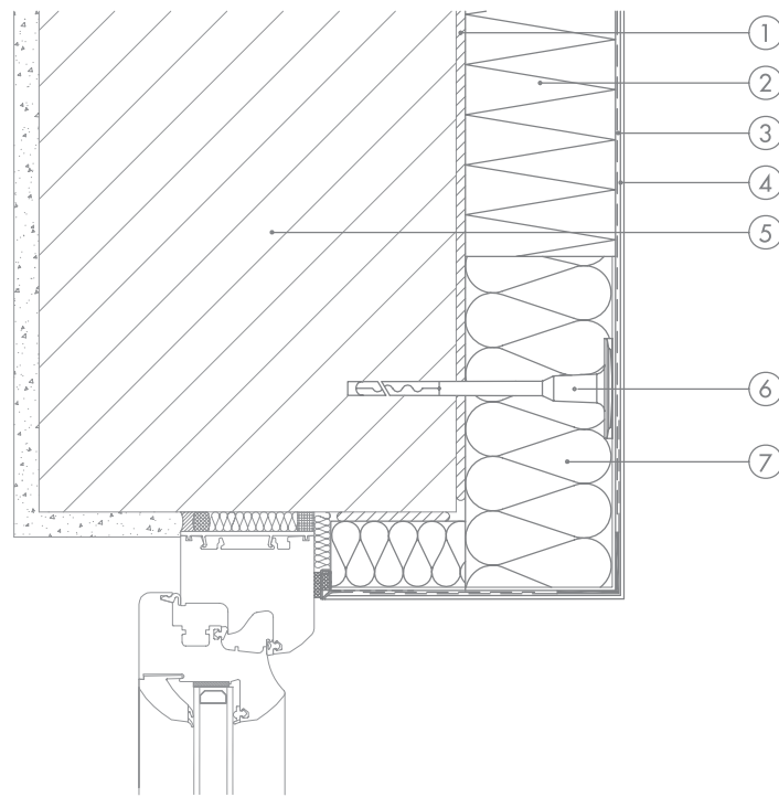
a) izvedba s izolacijom okvir
